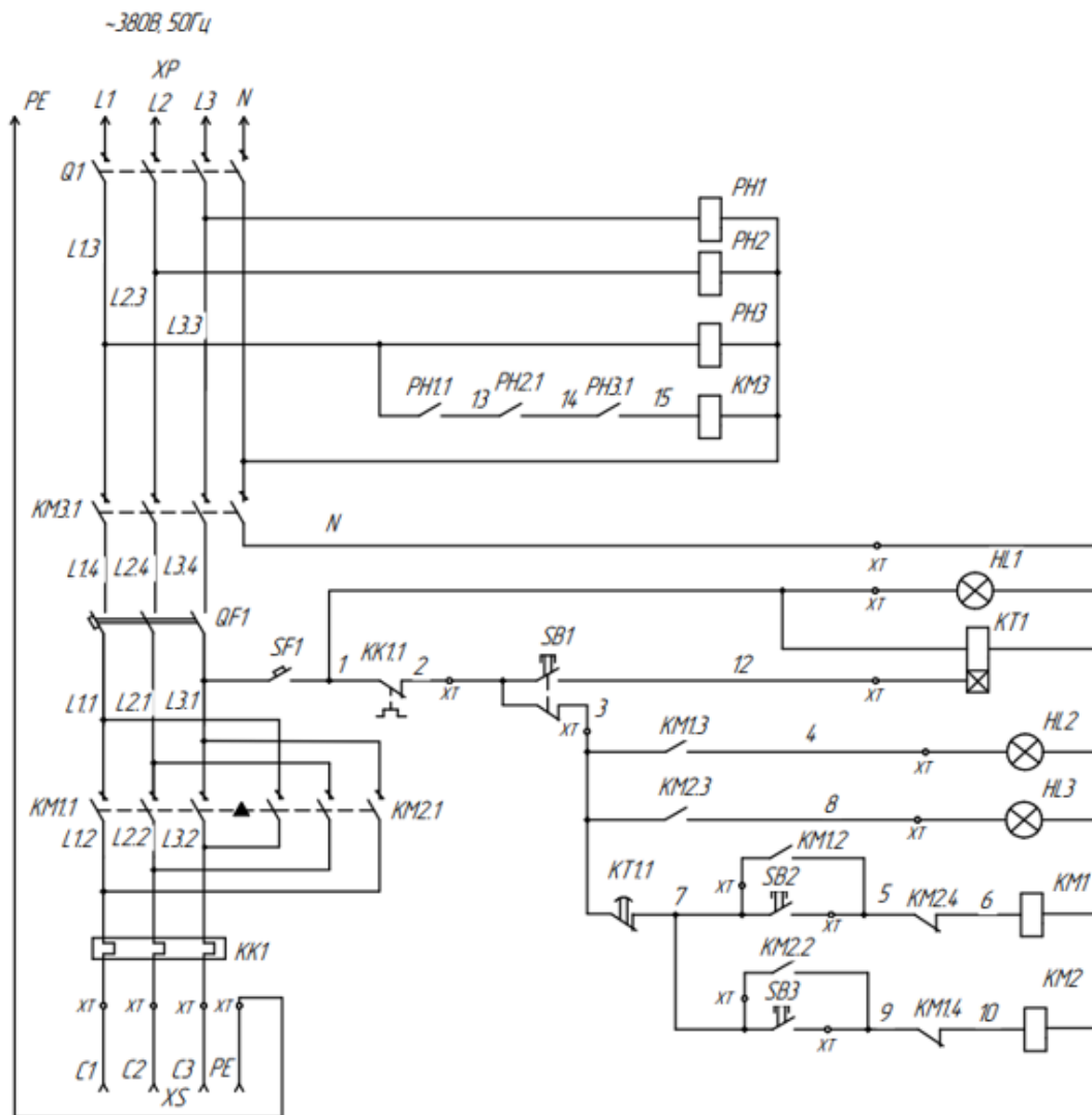
Схема электрическая принципиальная для ПУ
